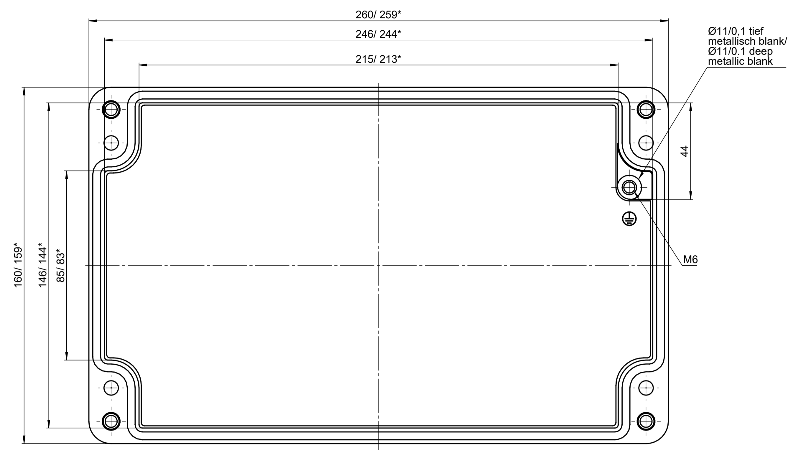
Deckel / Lid
