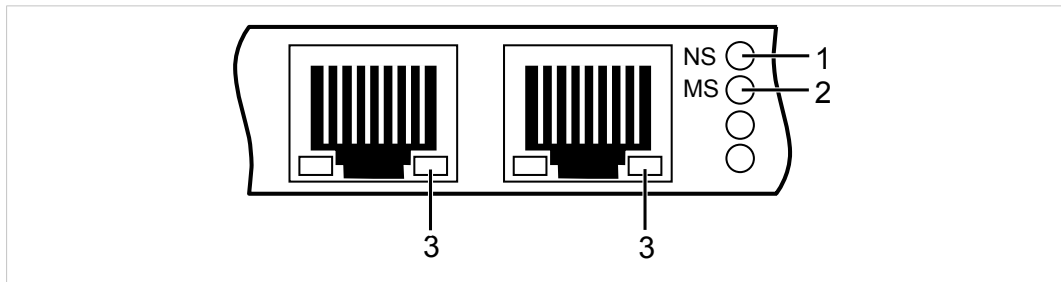
Fig. 11 LEDs Modbus
