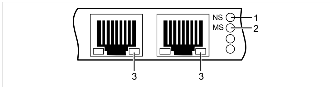
Fig. 10 LEDs PROFINET
