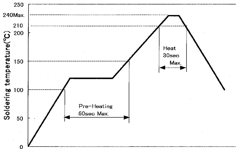
Fig.4 リフローソルダーリングの温度プロフィール
