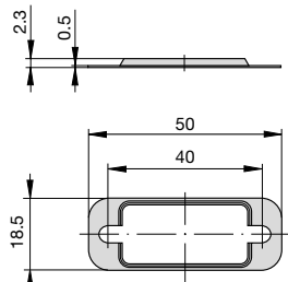
Fixing plate Y 301 056 02
