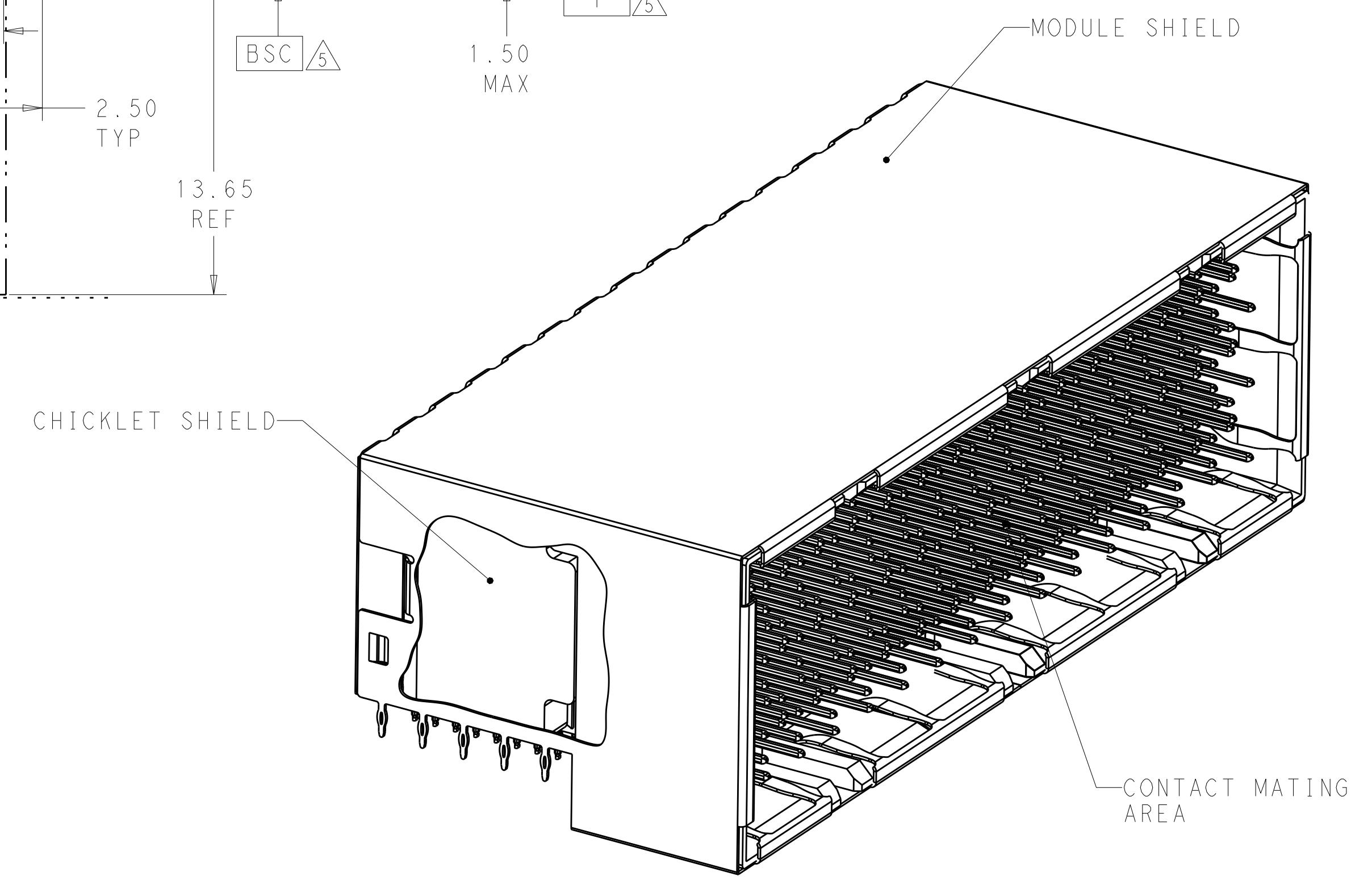
SCALE 4:1
