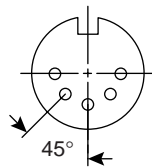
5 Pin 164-9350
