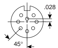
8 Pin 164-9380
