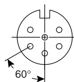
6 Pin 164-9360
