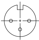
3 Pin 164-9330
