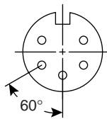
5 Pin 164-9351
