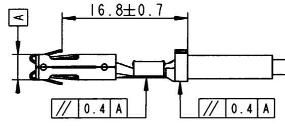
ANSCHLAGBILD FUER NORMALE ANWENDUNG CRIMPED TERMINAL NORMAL APPLICATION 2:1
