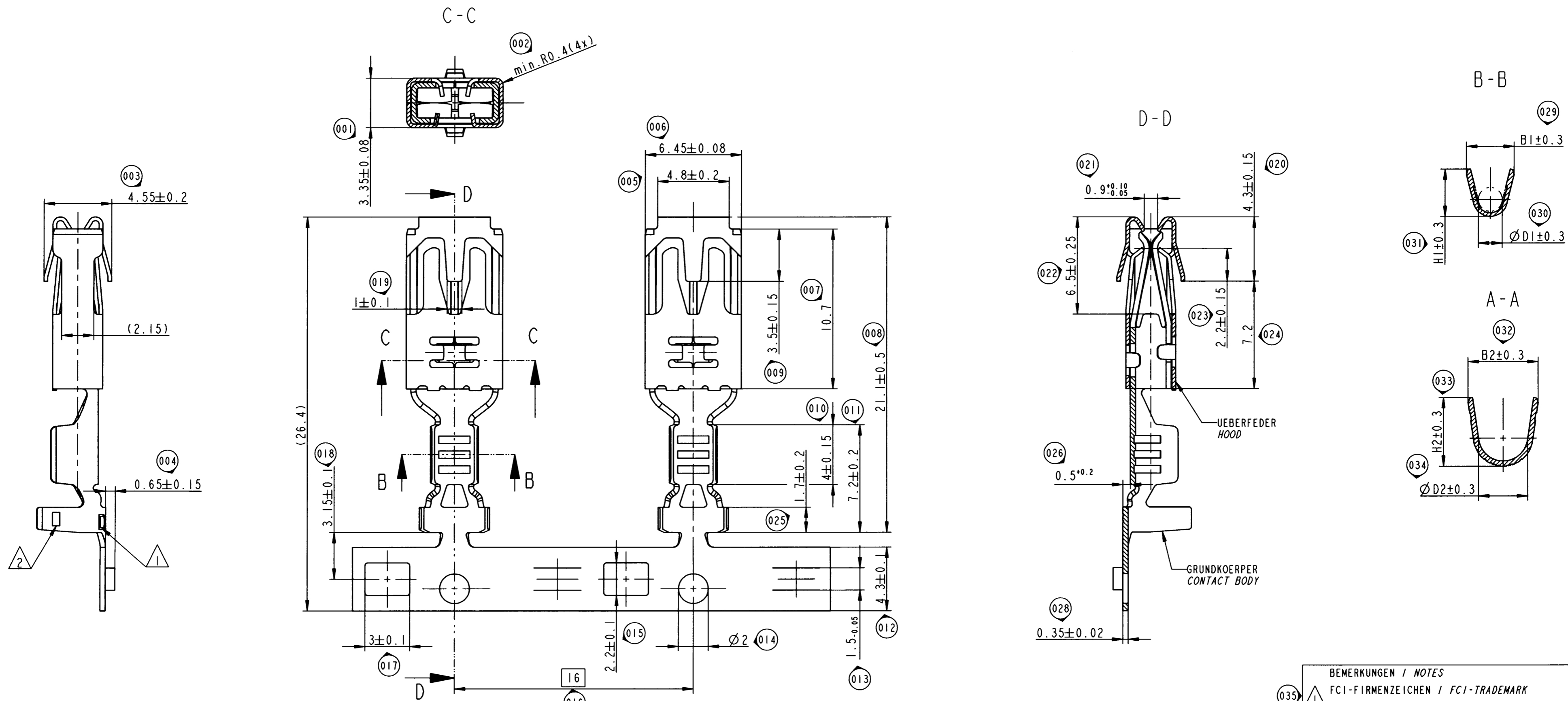
ANSCHLAGBILD MIT EINZELDICHUNG CRIMPED TERMINAL WITH SINGLE WIRE SEAL M 2:1
