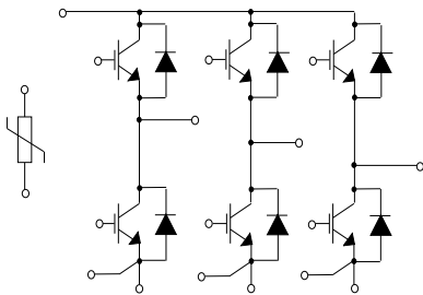
ACEPACK™ 2
