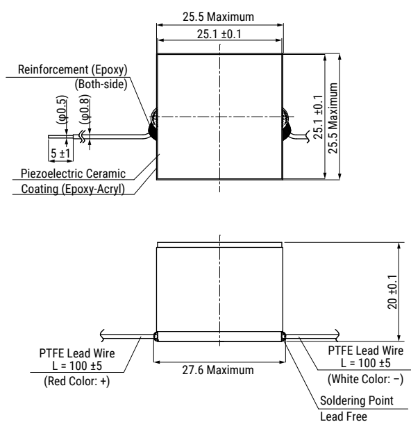
AE2525D15DF
