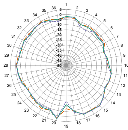
YZ-Plane Gain
