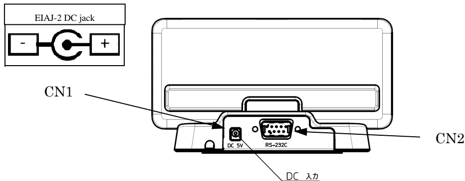
CN2 PIN 配置
