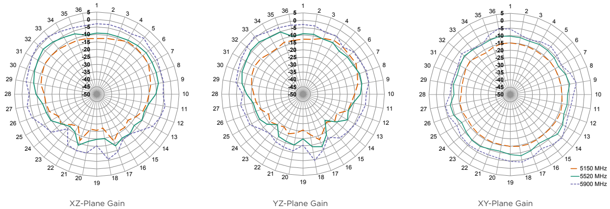
XZ-Plane Gain
