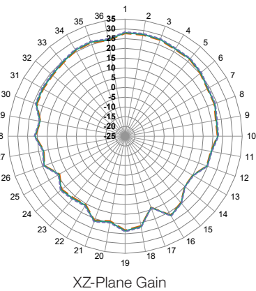
XZ-Plane Gain
