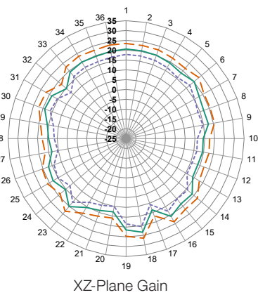
XZ-Plane Gain
