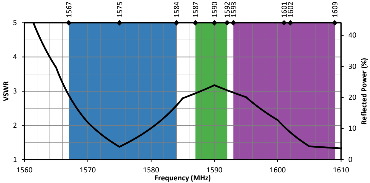
Figure 2. GNSSCP-TH18L1 VSWR
