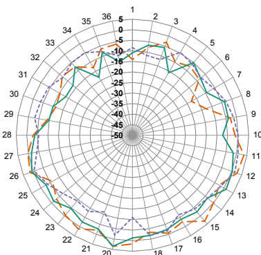
XZ-Plane Gain
