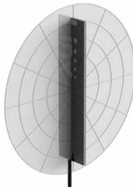
YZ-Plane Gain
