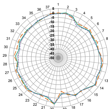
YZ-Plane Gain
