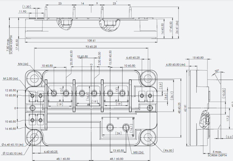
SP6LI
