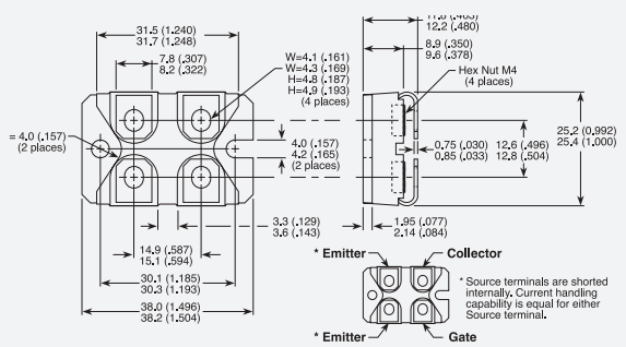
SOT-227
