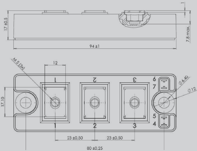
D1P
