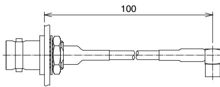
BNC(75)-BPJ-1.5CV-※
