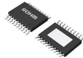
HTSSOP-B20
