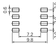
LAND PATTERNS (mm) 推奨ランド寸法
