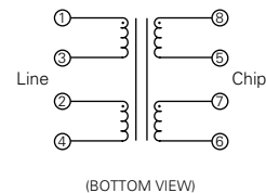
SCHEMATICS 結線図
