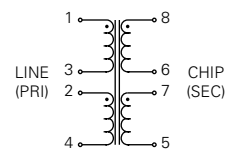
SCHEMATICS 結線図
