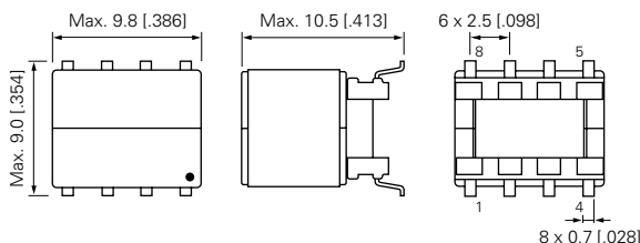
DIMENSIONS (mm) [ ] : inch 外形寸法図
