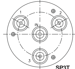
SP3T
