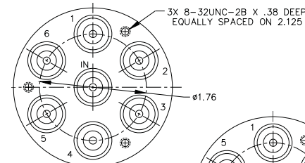
SP6T
