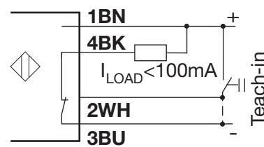
Fig. 7 NPN NC
