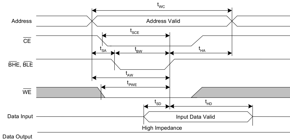
图 8. 第三个 SRAM 写周期 (受 \overline{BHE} 和 \overline{BLE} 控制) [28、29、30、31]
