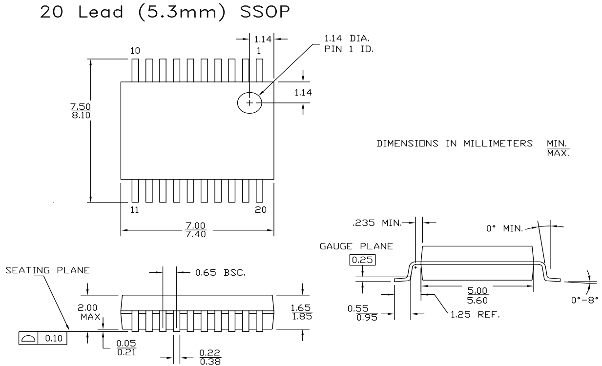
图 17. 20 引脚 SSOP (210 Mil) 封装外形 O20.21, 51-85077
