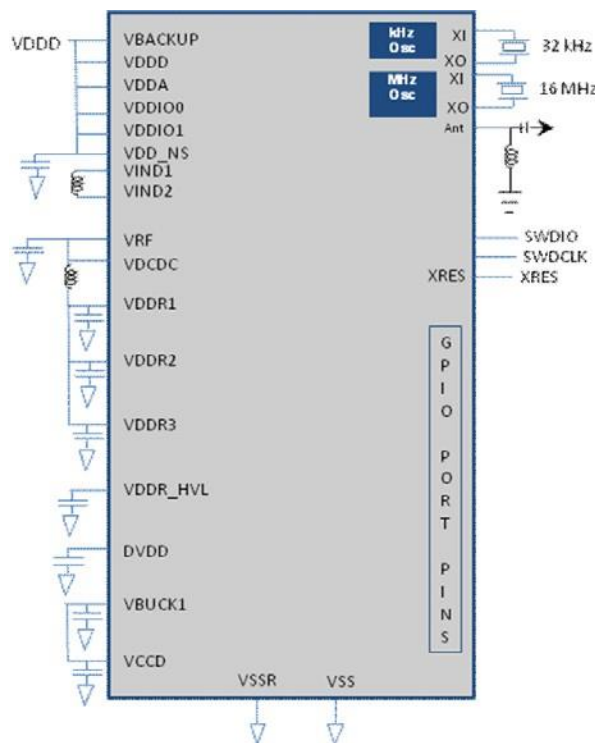
Figure 3. SOC 电源与无线连接 (用于 104-CSP 和 116-BGA 封装)
