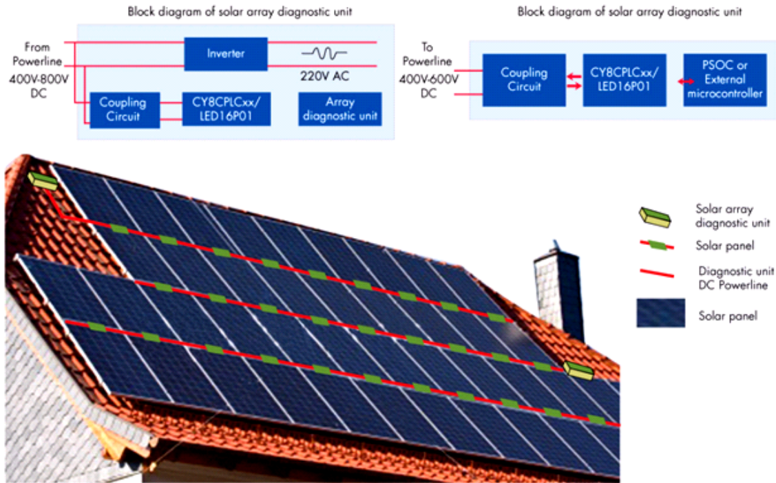
图 7. 智能能源管理（太阳能诊断）的电力线通信
