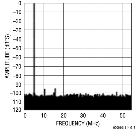
LTM9010-14: 8k Point FFT, f_{IN} = 5\text{MHz} , -1\text{dBFS} , 105\text{Mps}
