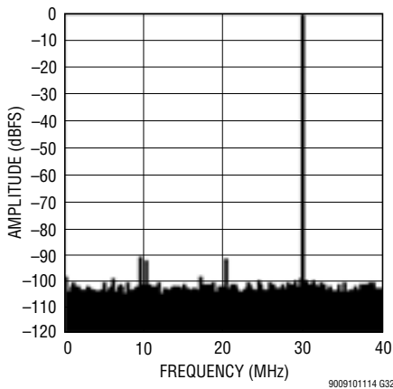
LTM9009-14: 8k Point FFT, f_{IN} = 30\text{MHz} , -1\text{dBFS} , 80\text{MSPS}
