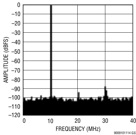
LTM9009-14: 8k Point FFT, f_{IN} = 70\text{MHz} , -1\text{dBFS} , 80\text{MSPS}
