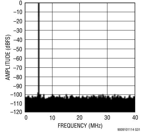
LTM9009-14: 8k Point FFT, f_{IN} = 5\text{MHz} , -1\text{dBFS} , 80\text{MSPS}
