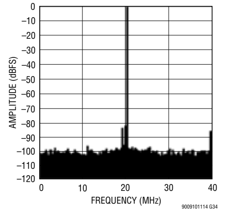
LTM9009-14: 8k Point FFT, f_{IN} = 140\text{MHz} , -1\text{dBFS} , 80\text{MSPS}
