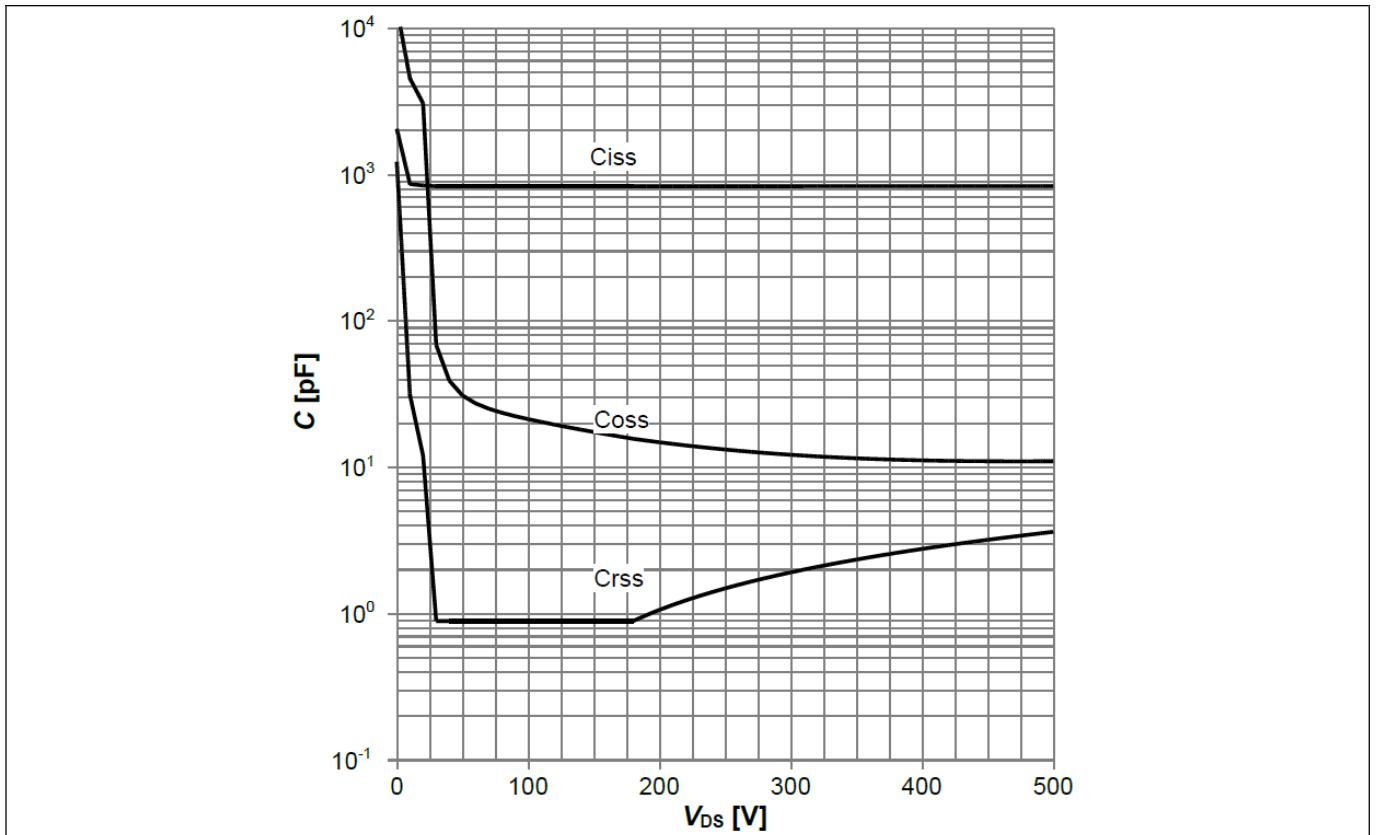
图 33 ICE5AR0680AG 的典型 CoolMOS™ 电容 (C=f(V DS ); V GS =0 V; f=250 kHz)
