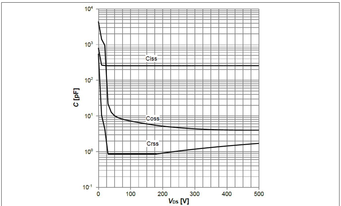
图 32 ICE5GR1680AG 的典型 CoolMOS™ 电容 (C=f(V DS ); V GS =0 V; f=250 kHz)
