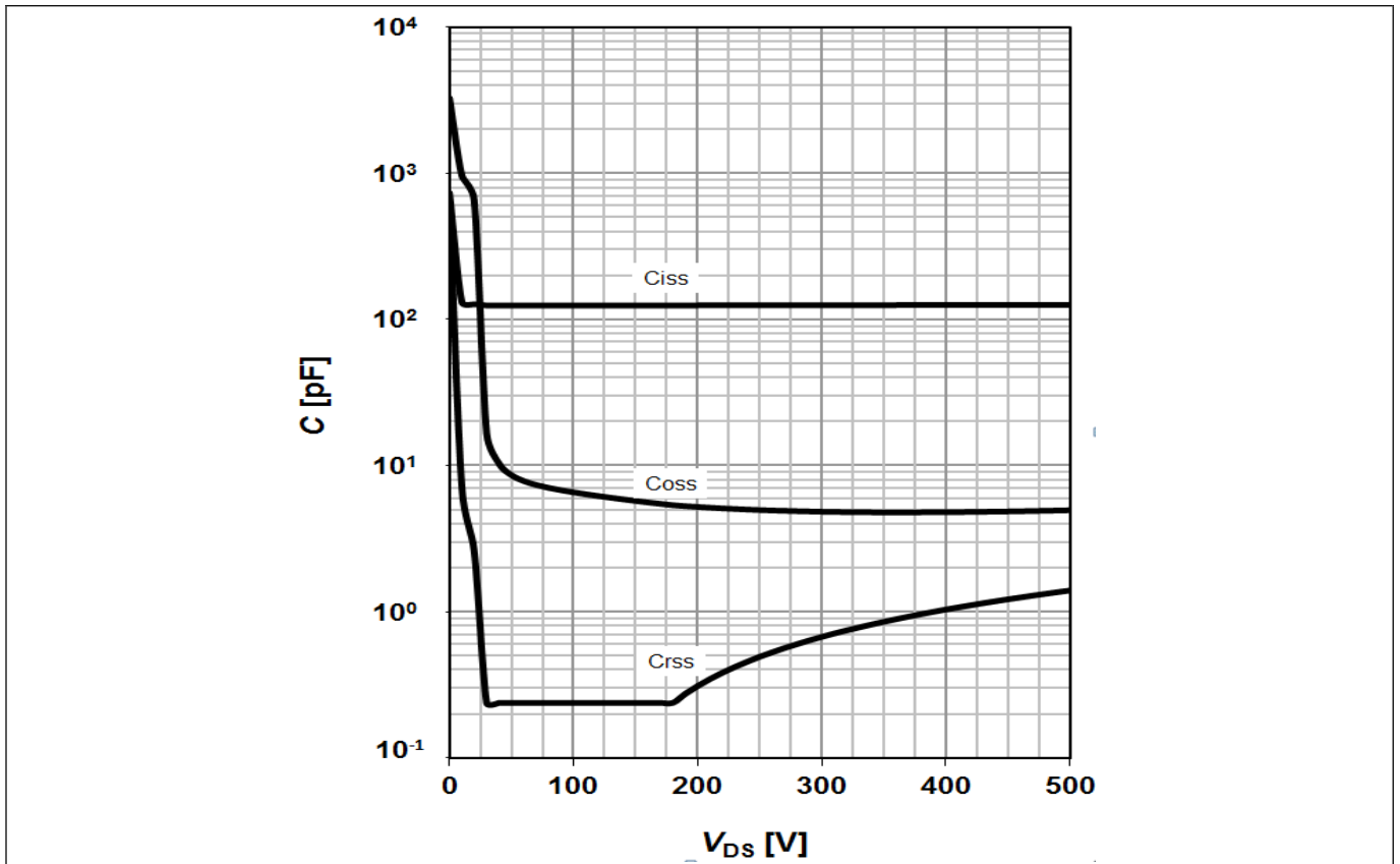
图 31 ICE5GR2280AG 的典型 CoolMOS™ 电容 (C=f(V DS ); V GS =0 V; f=250 kHz)
