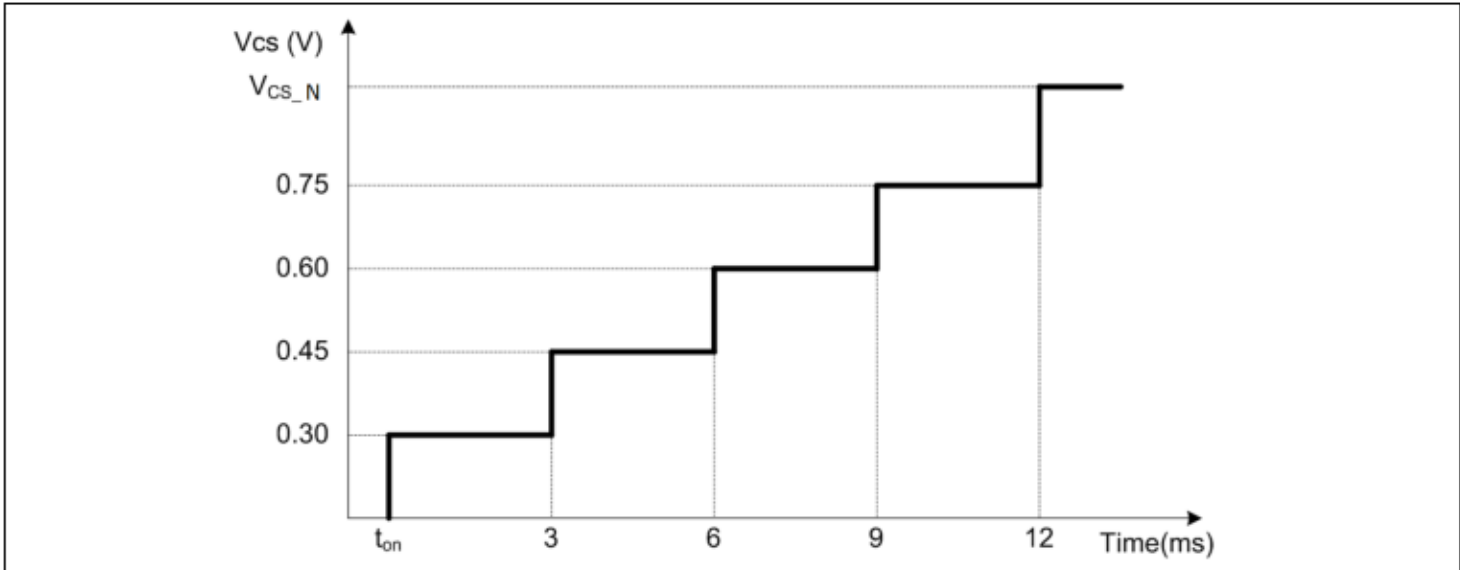
图 6 软启动期间的最大电流感测电压
