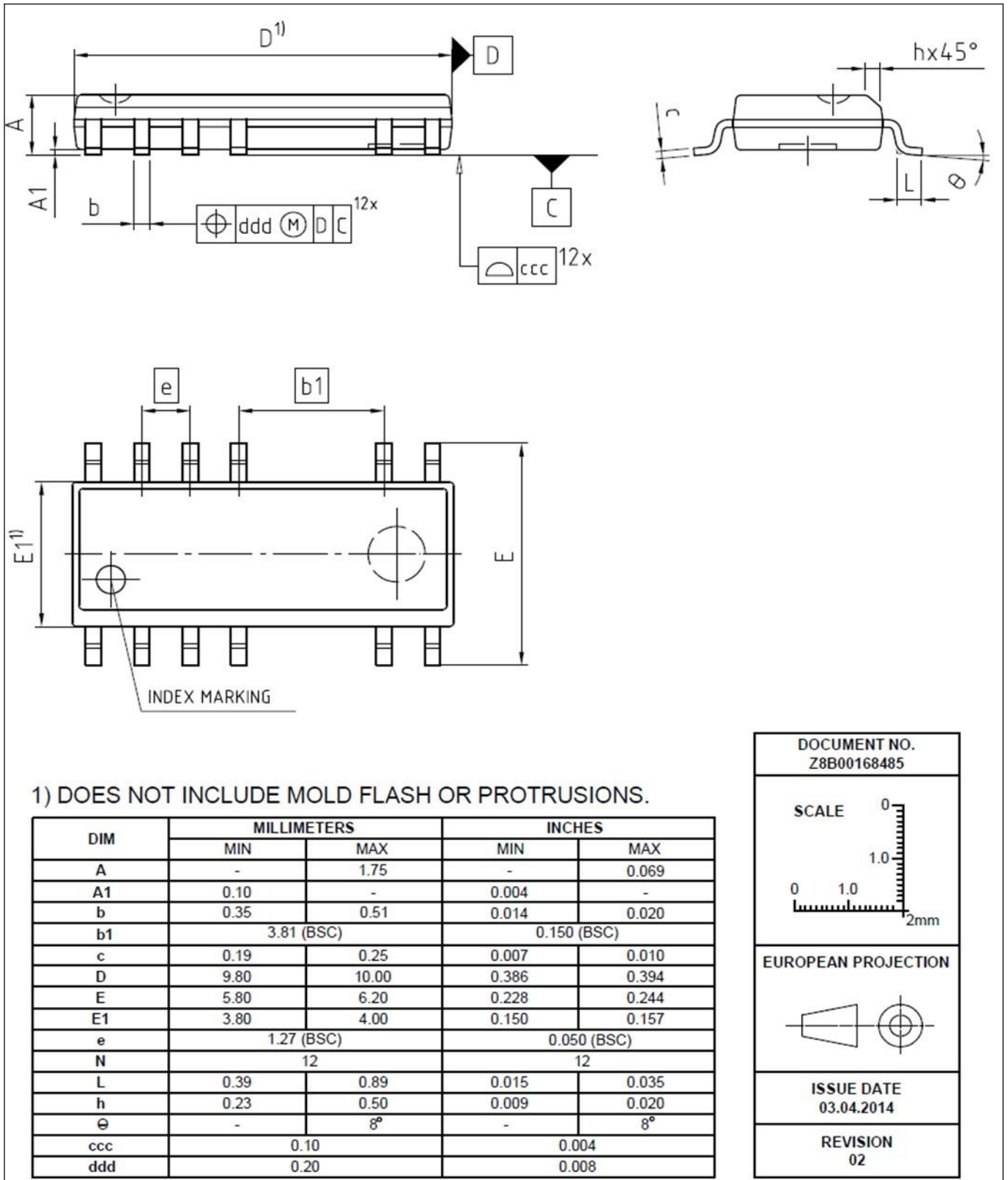
图 39 PG-DSO-12
