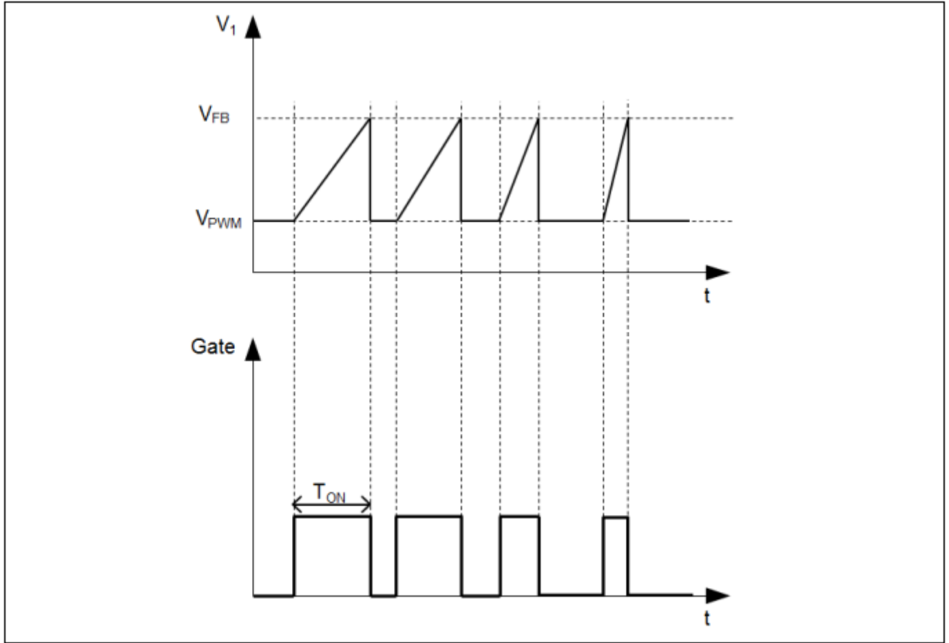
图7 脉宽调制
