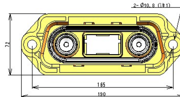
Receptacle
