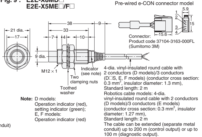
Fig. 9 : E2E-X8MD□ E2E-X5ME□/F□
