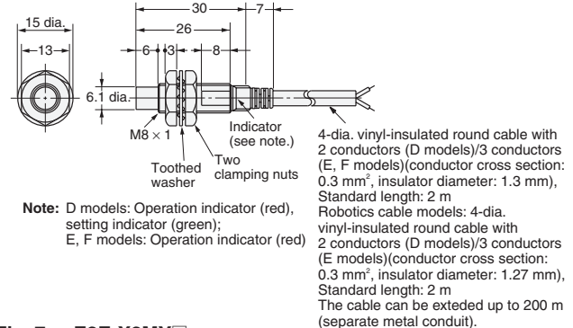
Fig. 7 : E2E-X2MY□
