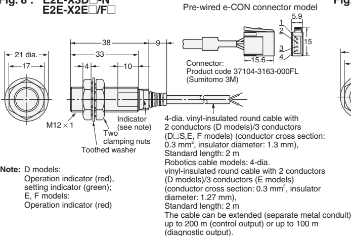
Fig. 8 : E2E-X3D□-N E2E-X2E□/F□
