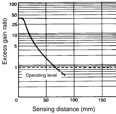
E32-TC200F/TC200F4 with E3X-A11 amplifier
