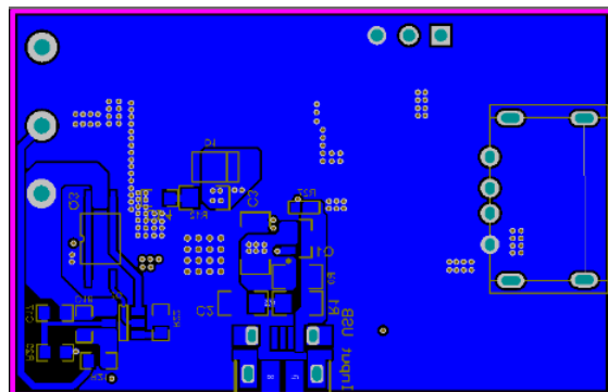
Bottom Layer
