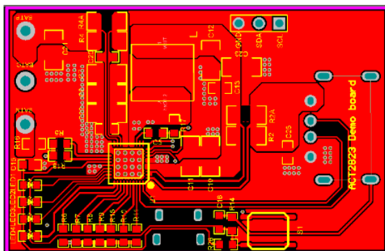
TOP Layer
