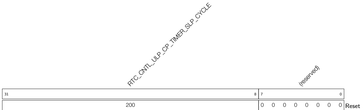
Register 1.2: RTC_CNTL_ULP_CP_TIMER_1_REG (0x0130)
