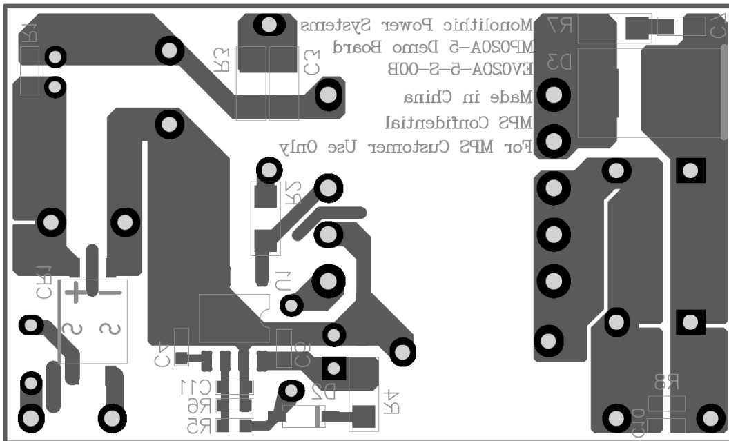
Figure 3—Bottom Layer
