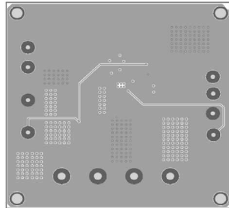
Figure 4— Inner 2 Layer
