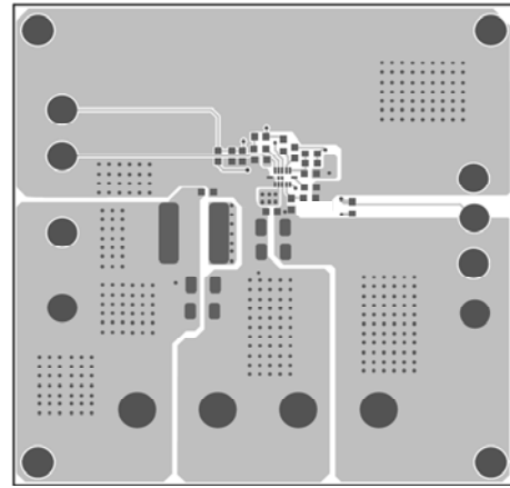
Figure 2—Top Layer
