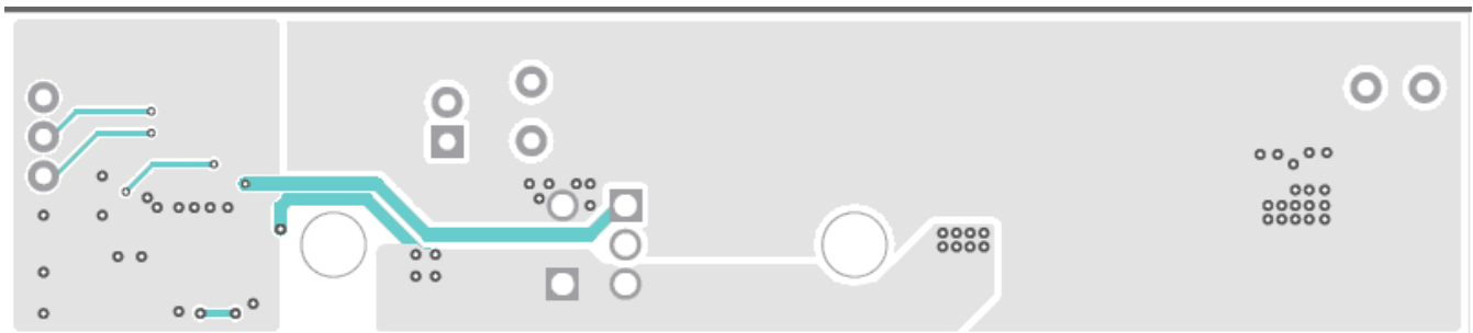
Figure 4—Bottom Layer
