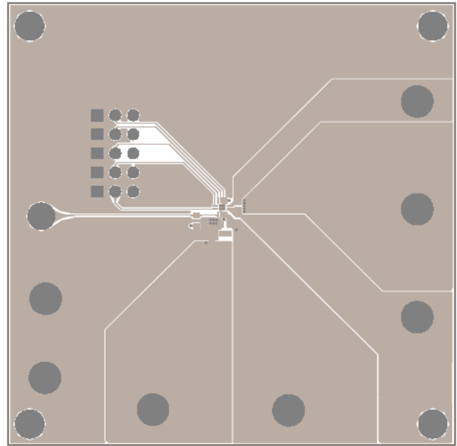
Figure 5—Top Layer
