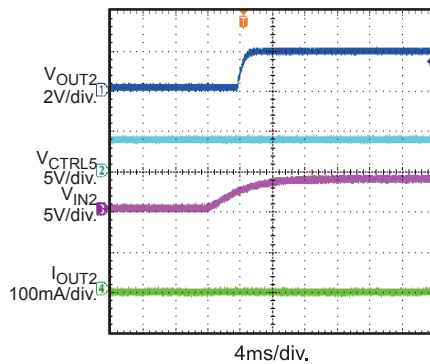
VIN On
