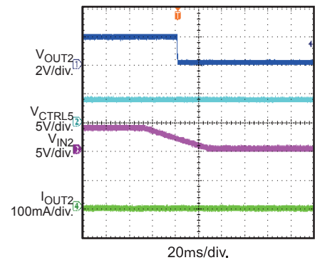
VIN Off
