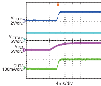
VIN On
