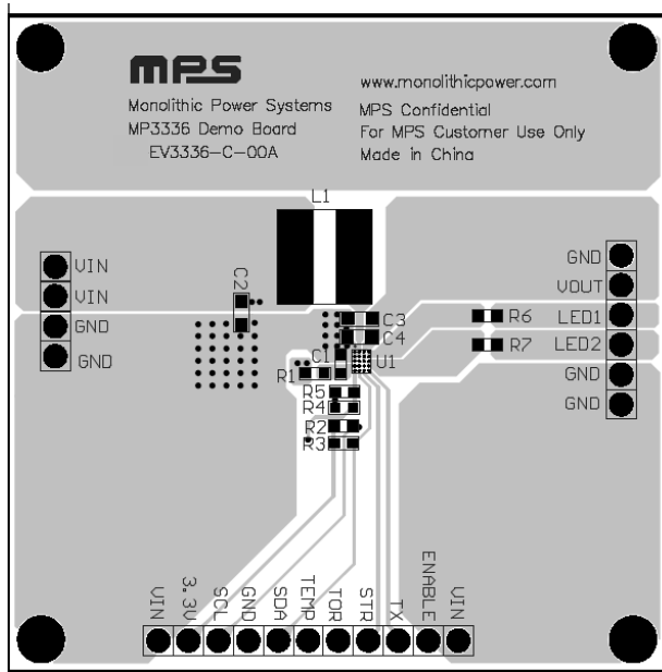
Figure 1—Top Layer
