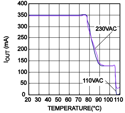
NTC Curve NTC=220kΩ
