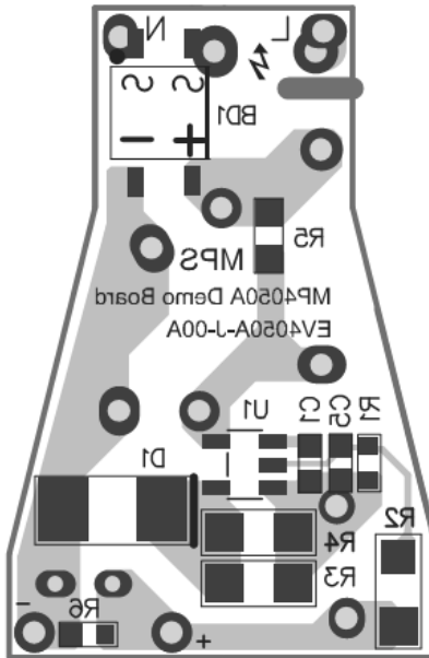
Figure 3—Bottom Layer
