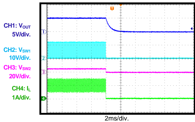
EN Pin Disable Load = 1A
