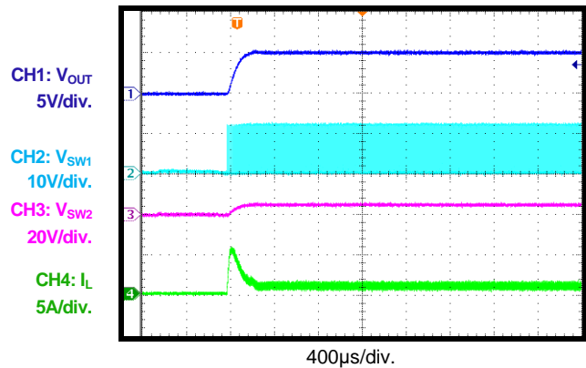
EN Pin Enable Load = 1A
