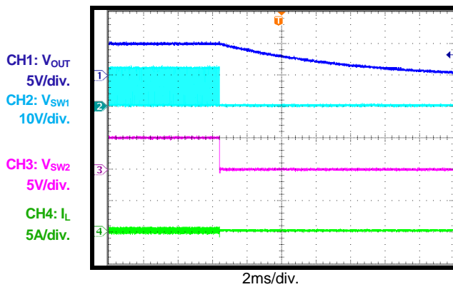
EN Pin Disable Load = 0A
