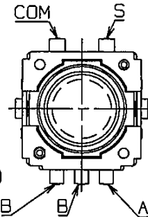
(ENCODER)
