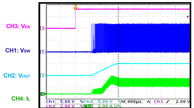
En On I_{OUT} = 2A
