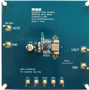
LxWxH (8.3cmx8.3cmx1.3cm)
