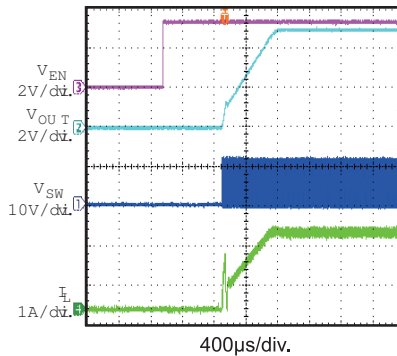
En On I_{OUT} = 2A
