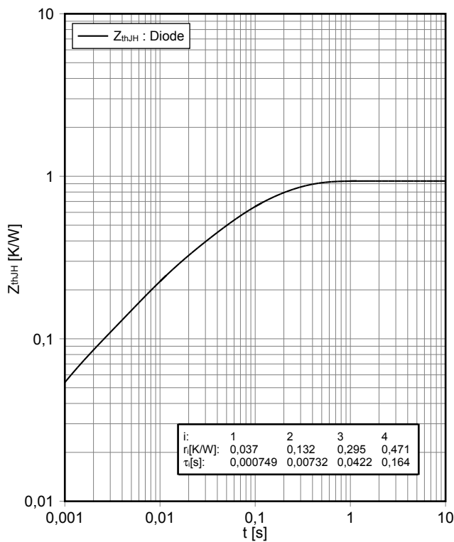
瞬态热阻抗 二极管, D2 / D3 transient thermal impedance Diode, D2 / D3
