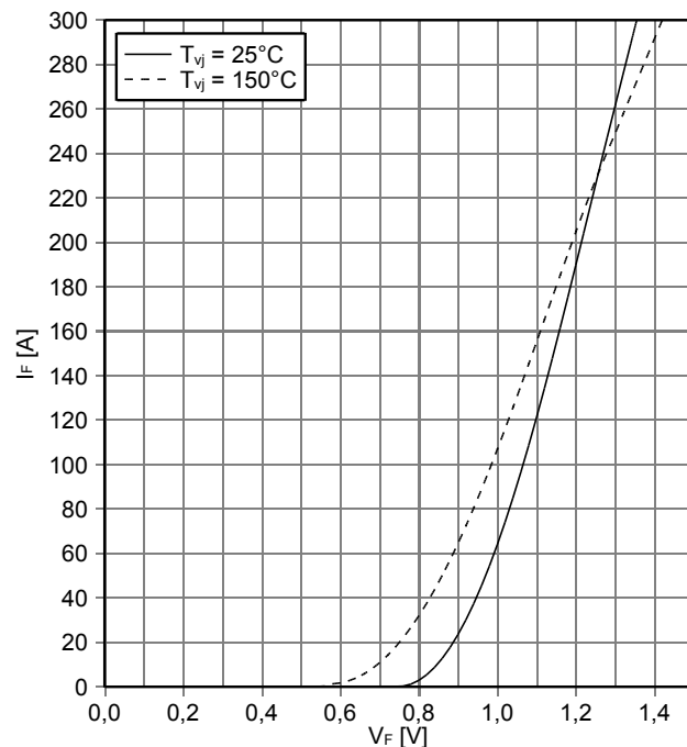
順方向特性 Diode、整流器 (典型) forward characteristic of Diode, Rectifier (typical)
