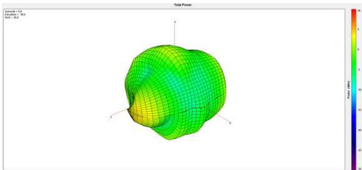
2100MHz
