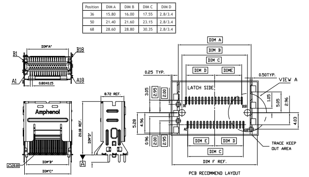
Drawing for mini SAS
